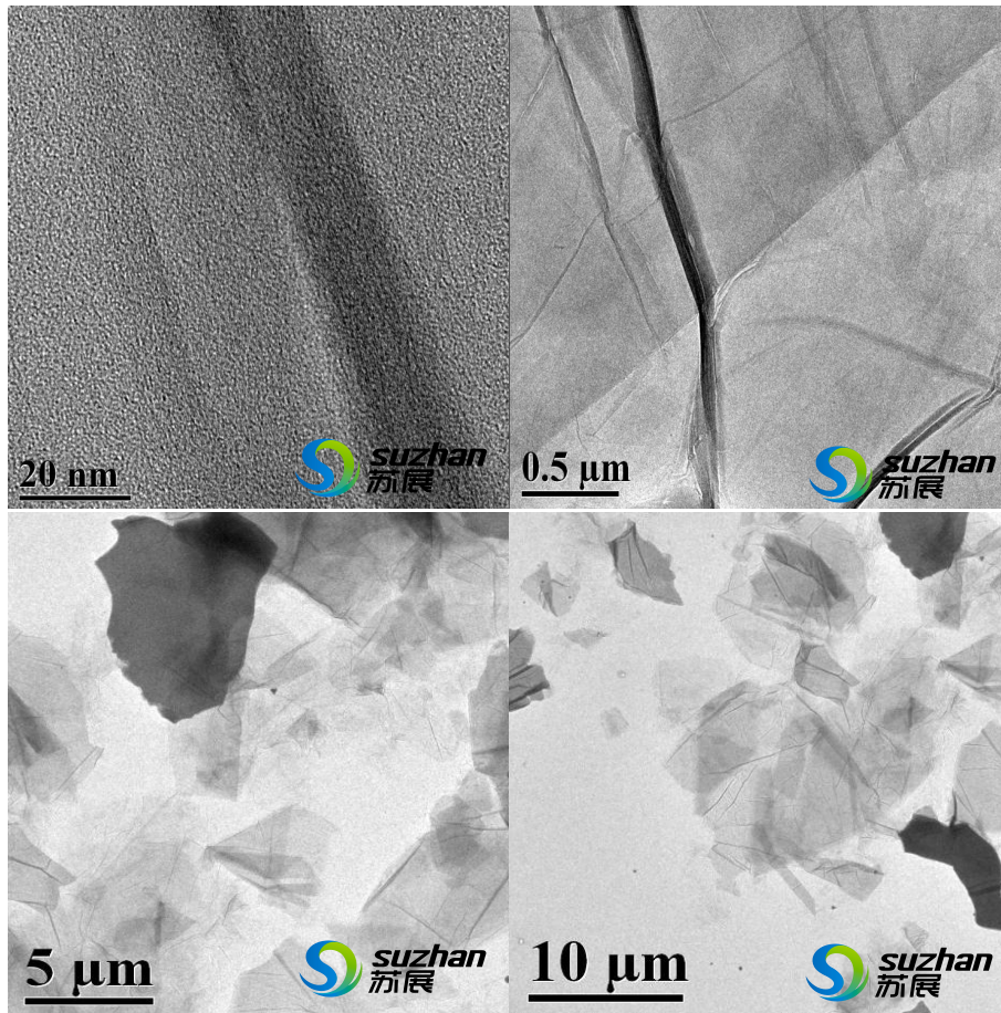
图2 工业级氧化石墨烯的TEM图
