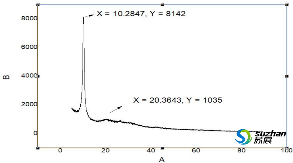
图 1 工业级氧化石墨烯的 XRD 图
